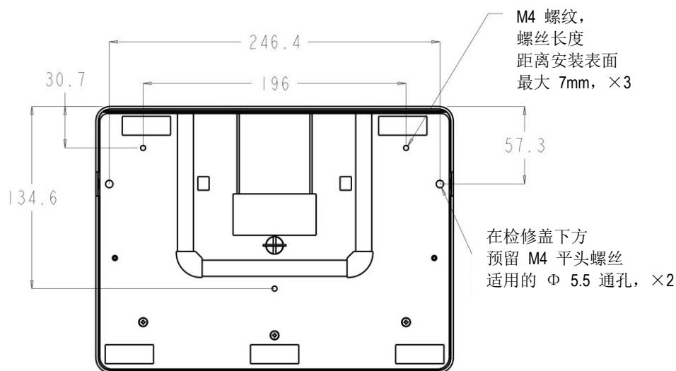
1517 支架仰视图
