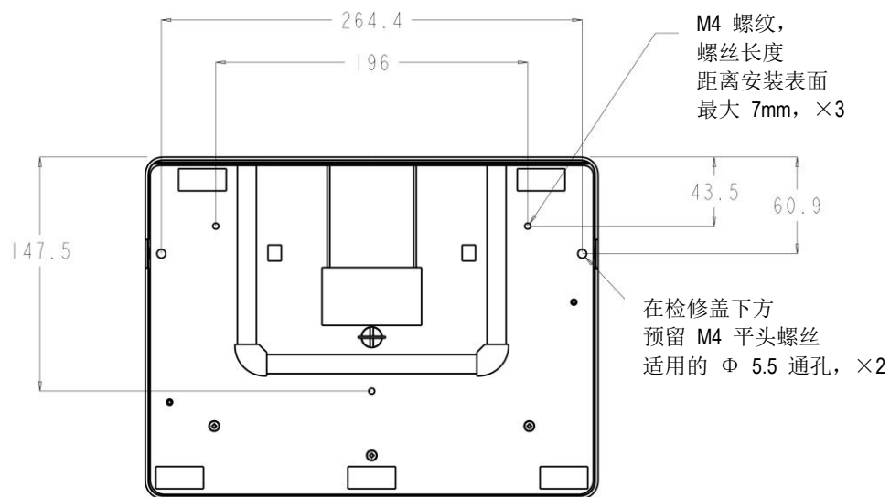
1717 支架仰视图
