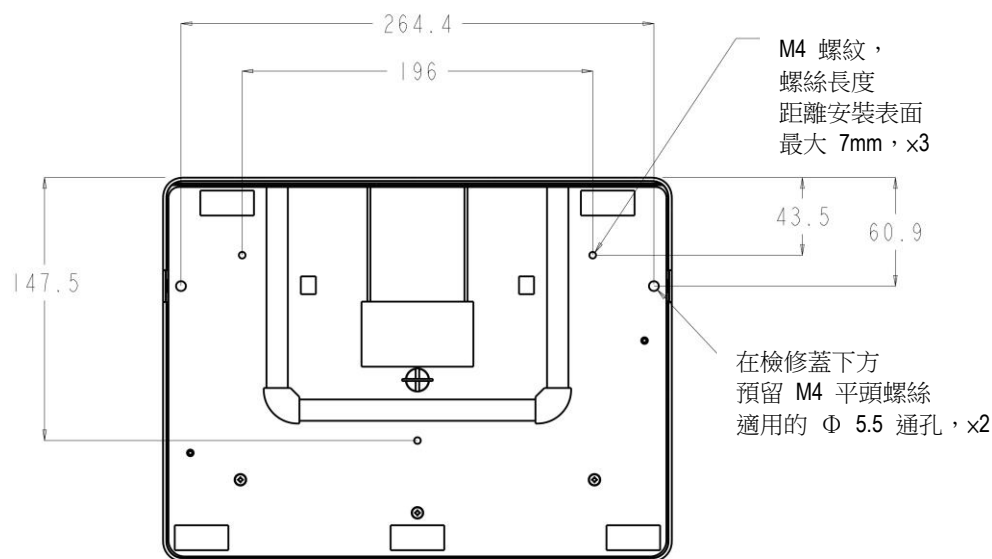
1717 支架仰視圖
