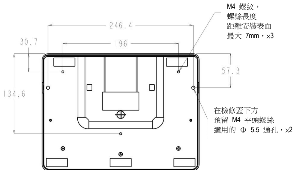
1517 支架仰視圖
