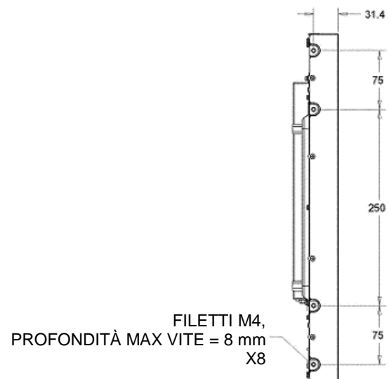
MONTAGGIO LATERALE VERTICALE (SINISTRA/ DESTRA)
