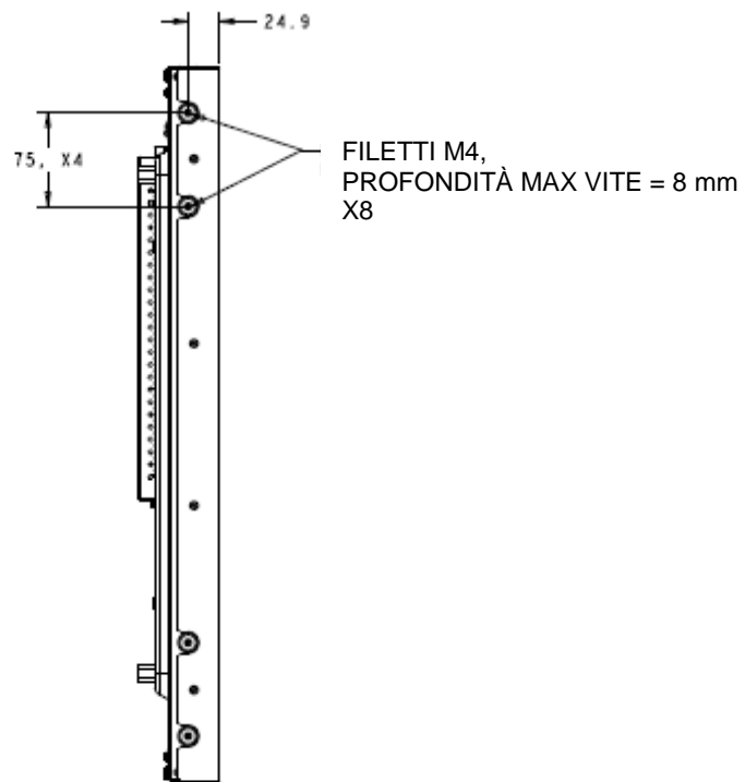
MONTAGGIO LATERALE VERTICALE (SINISTRA/ DESTRA)
