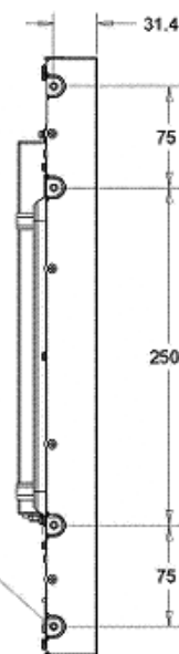
ВЕРТИКАЛЬНЫЙ БОКОВОЙ МОНТАЖ (СЛЕВА/СПРАВА)
