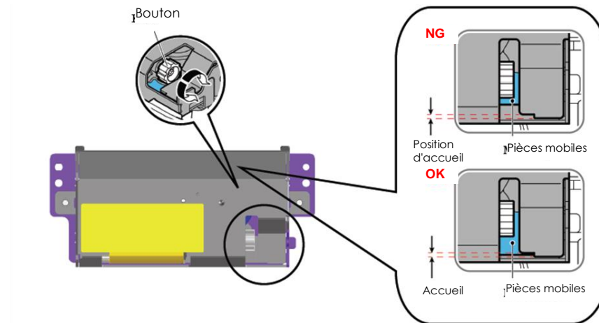
Figure 6. En cas de bouchage papier, faites tourner le bouton pour éliminer le bouchage papier.
