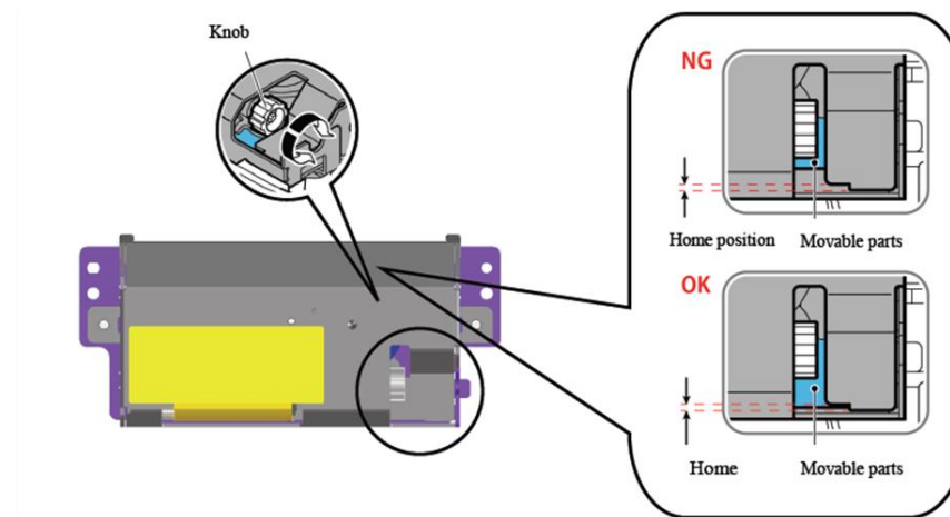
Figura 6. In caso di inceppamento della carta, ruotare la manopola per rimuovere la carta.
