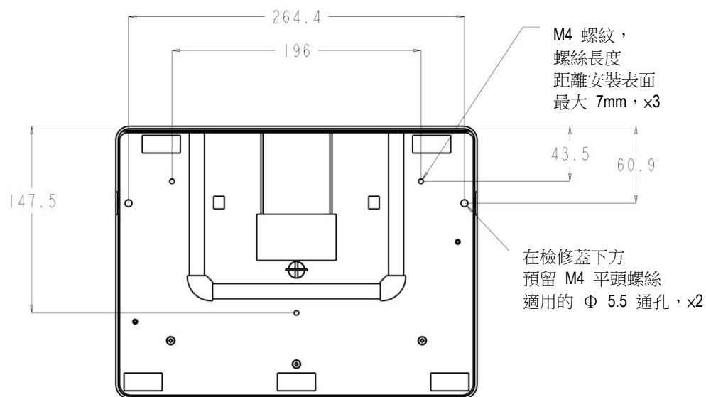
1717 支架仰視圖
