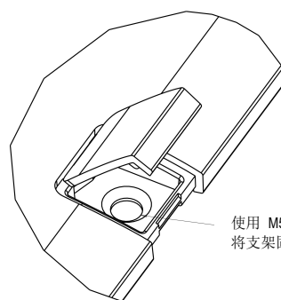
详图 A 比例 3.000
