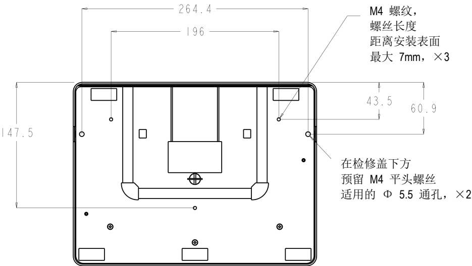
1717 支架仰视图
