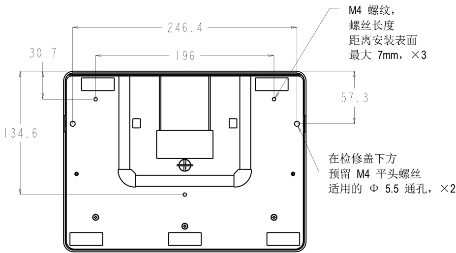
1517 支架仰视图
