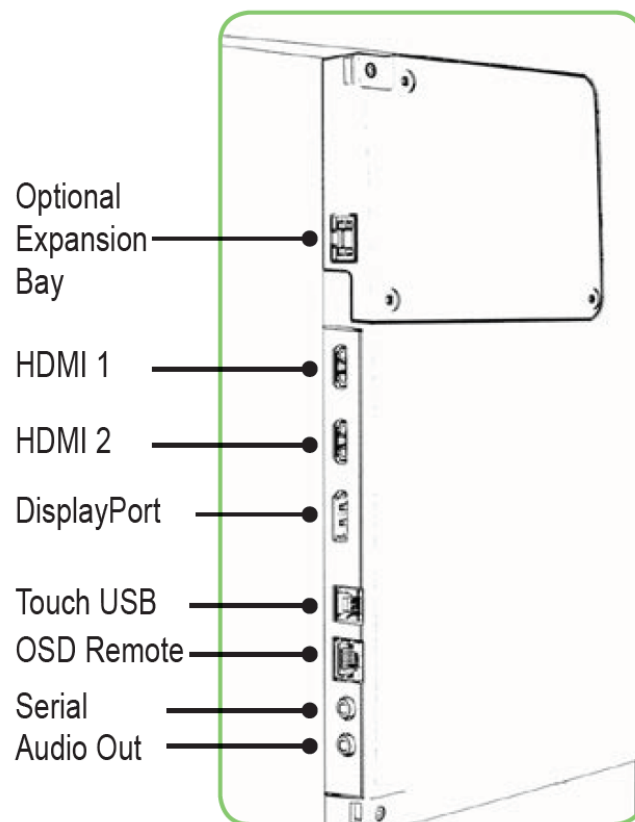
Изображение доступных портов ввода/вывода на мониторе
